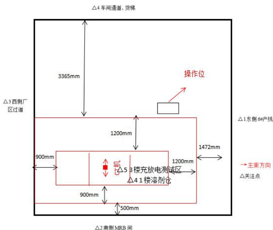
图 11-1 工业 CT 机的摆放位置图
